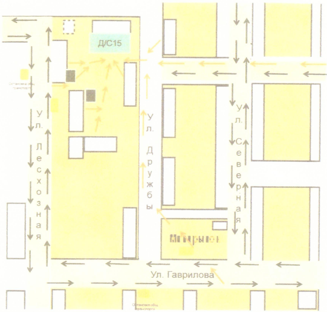
1.2. Схема организации дорожного движения в непосредственной близости от образовательного учреждения с размещением соответствующих технических средств, маршруты движения детей и расположение парковочных мест автотранспорта
